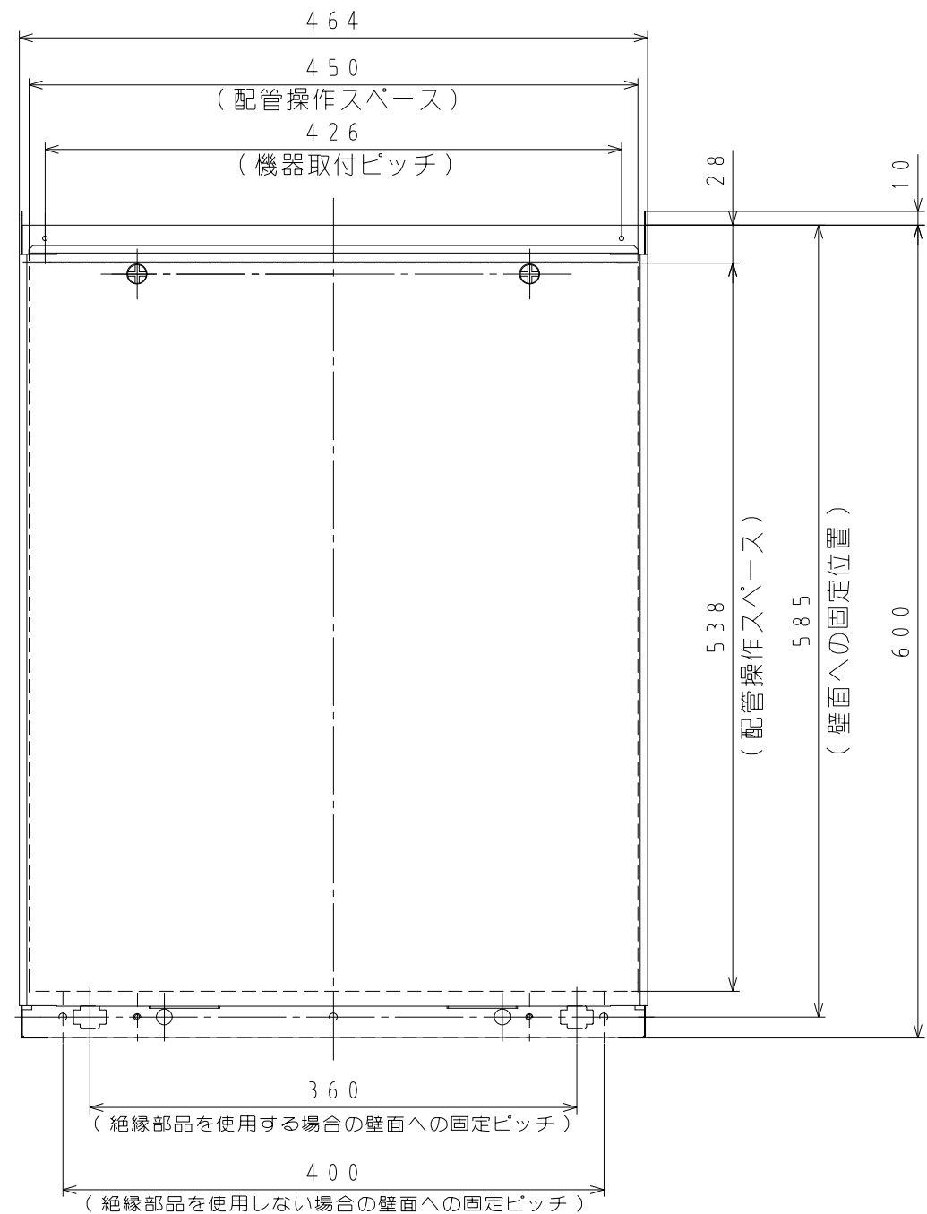
① 寸法図（単位：mm）
