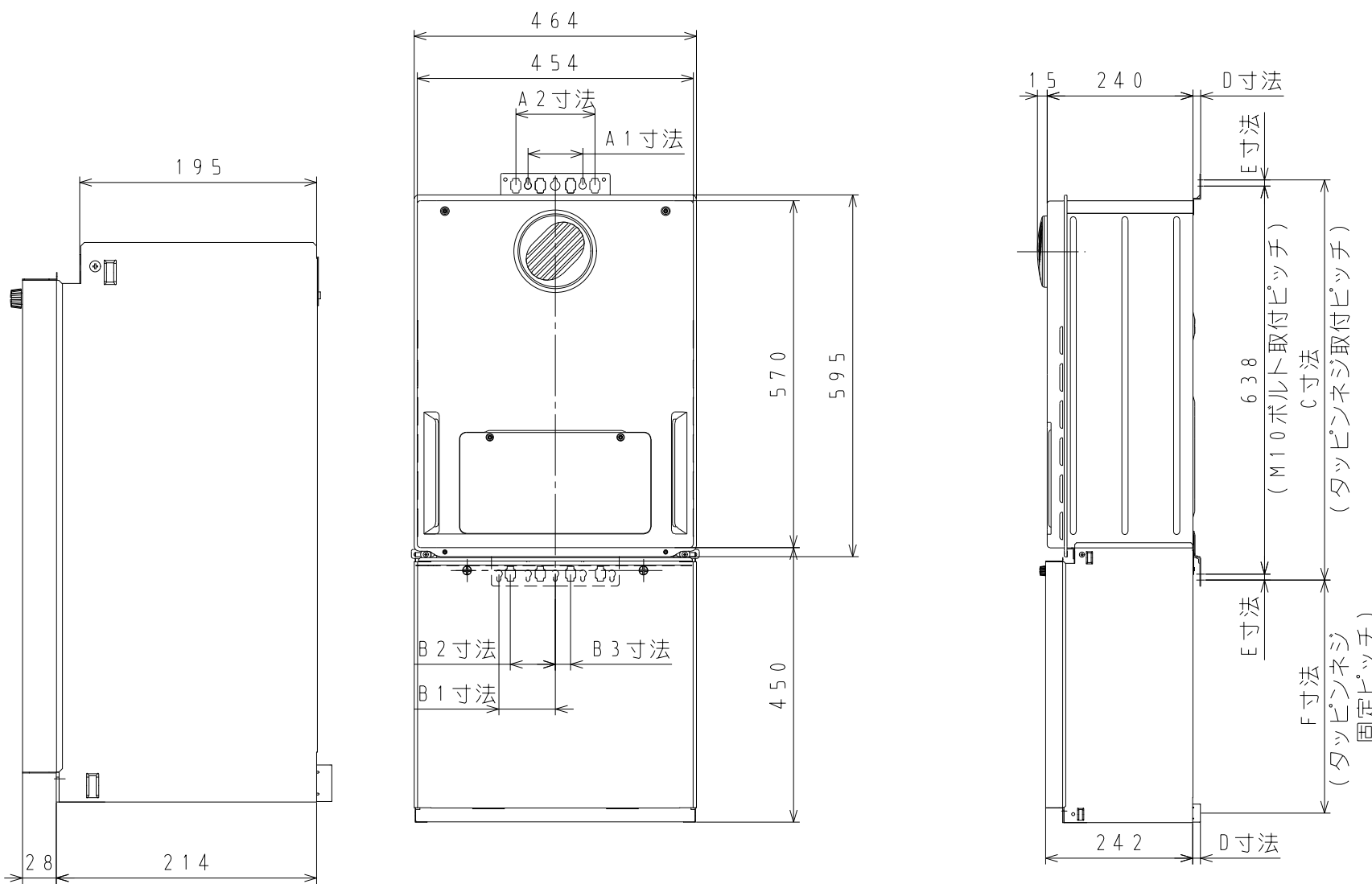
② XT4219KRSAWCM取付け寸法図
