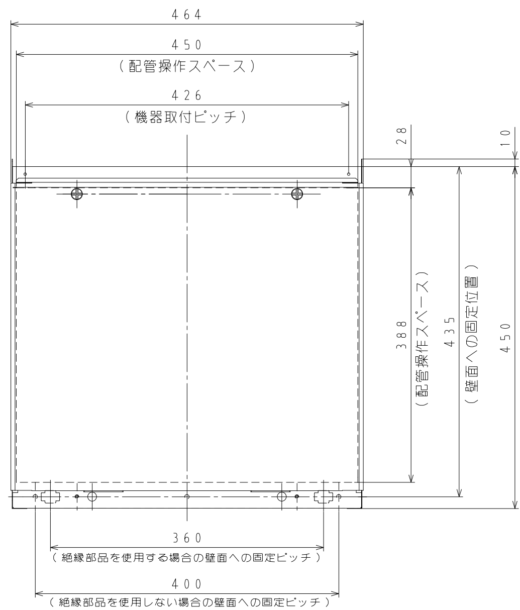
① 寸法図（単位：mm）
