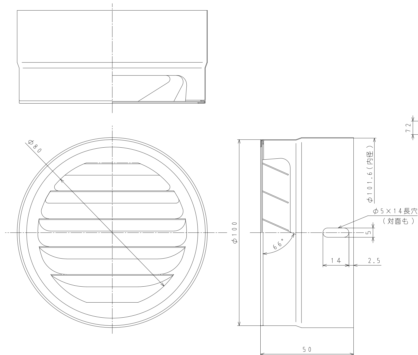
①本体寸法図(単位:mm)
