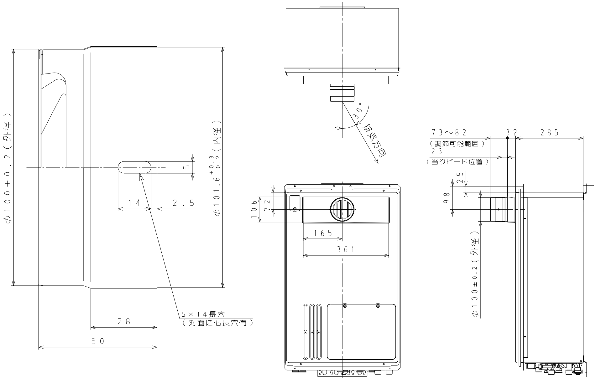
② GH-SD2700ZTH の場合 取付寸法図(単位:mm) (図は右吹出しを示す)
