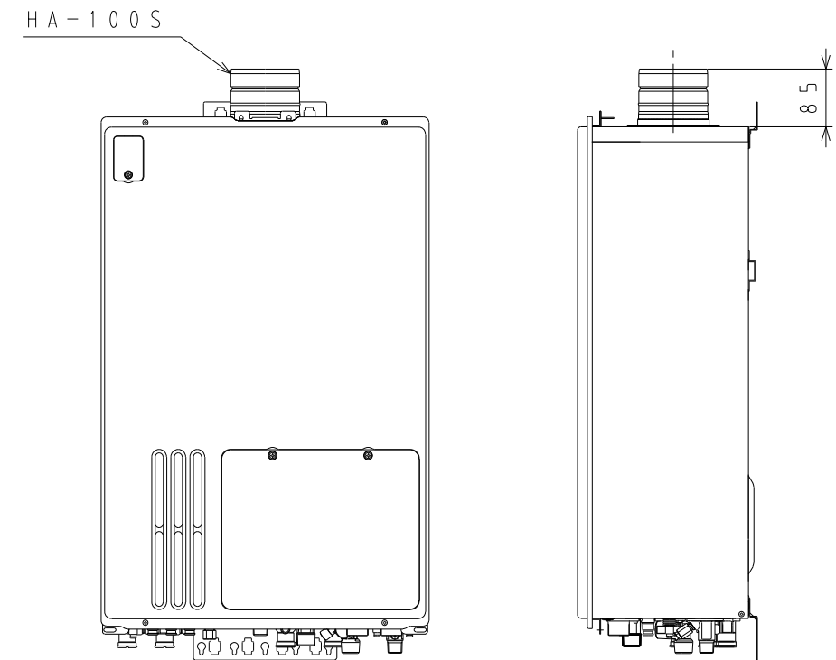
2 . X T 4 2 1 2 A R S 9 A W 3 T 設置例
