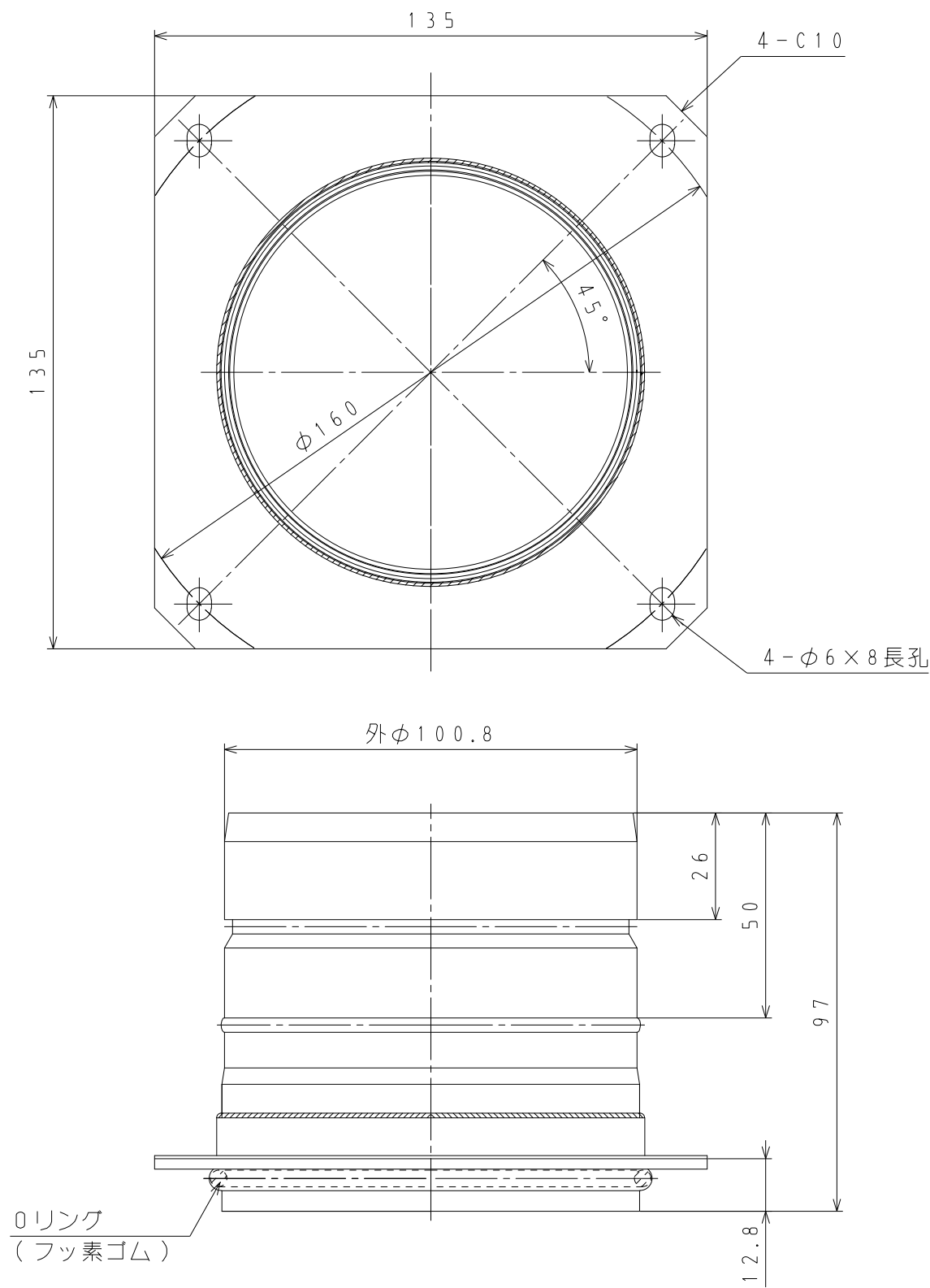
1 . 本体寸法図 ( 単位 : mm )
