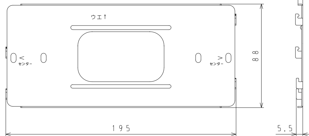
壁取付金具 寸法図
